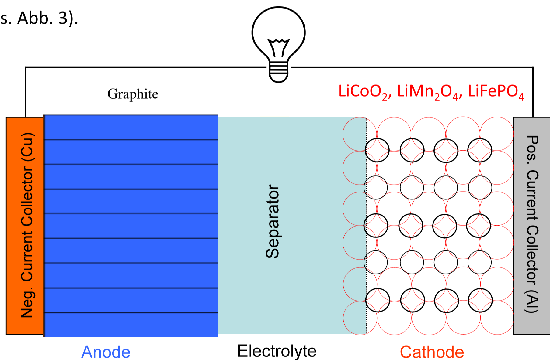
Abb. 2: Darstellung einer gewöhnlichen LIB
