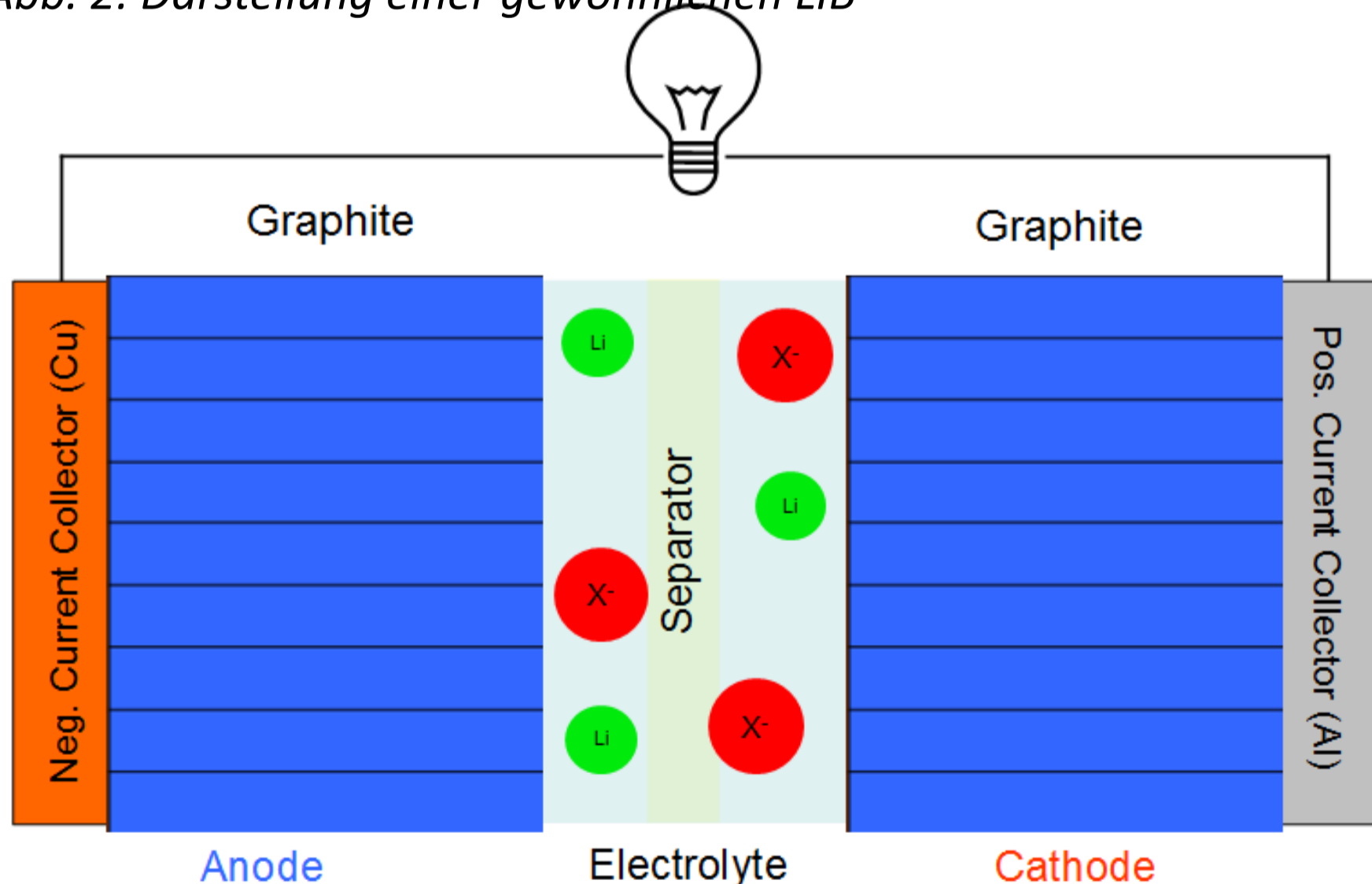
Abb. 2: Darstellung einer gewöhnlichen LIB
