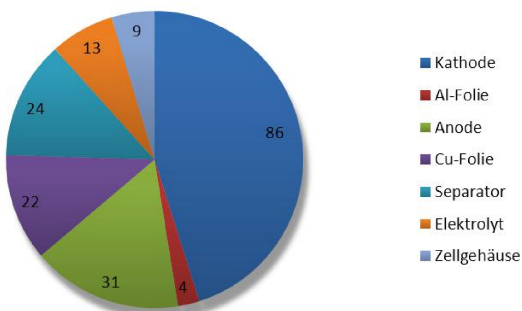
Abb. 1: Kostenverteilung (in €/kWh) einer LIB
