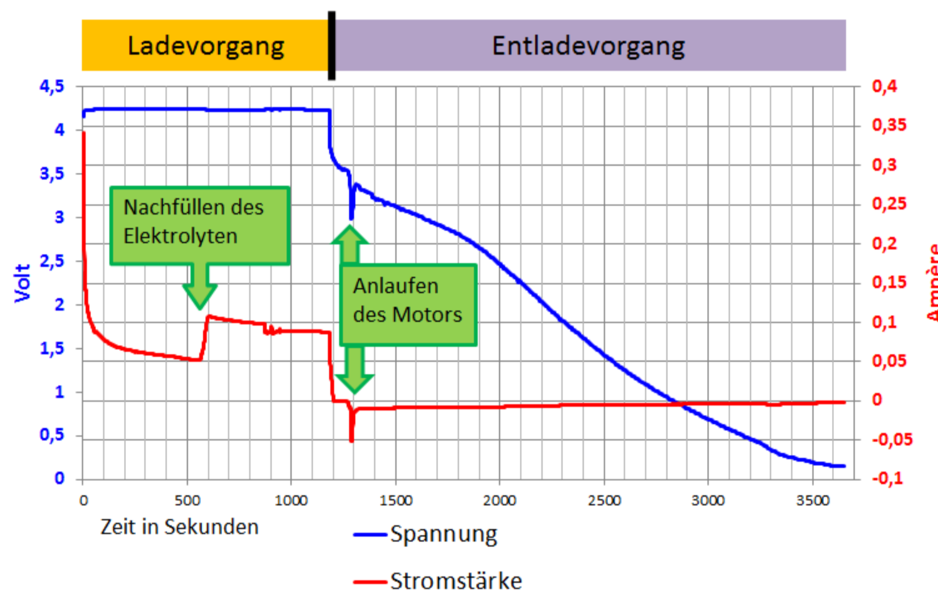
Abb. 4: Zyklus eines Akkus (geladen mit 4,2 V)
